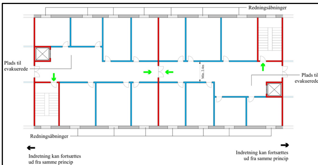
Figur 2.3.9 Præ-accepteret løsning for vandret evakuering fra et sengeafsnit på et hospital.
