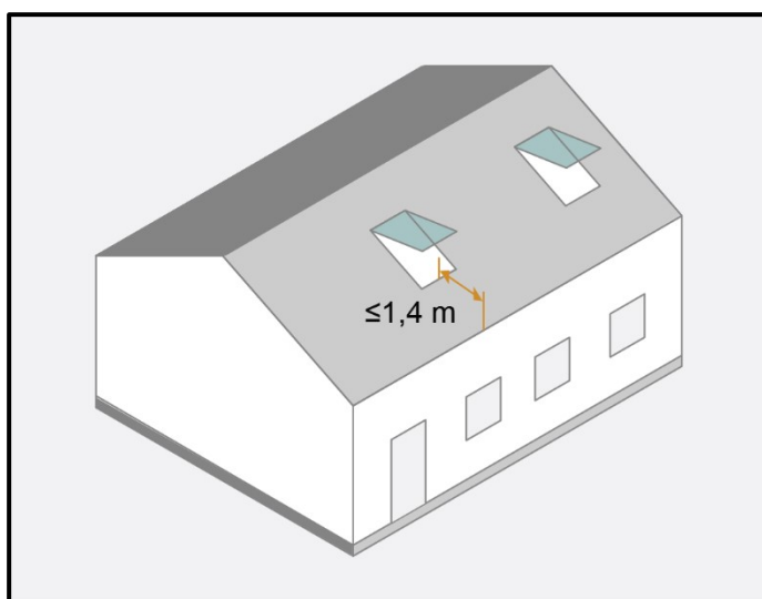
Figur 2.4.2 Udformning af redningsåbning i tagflade.
