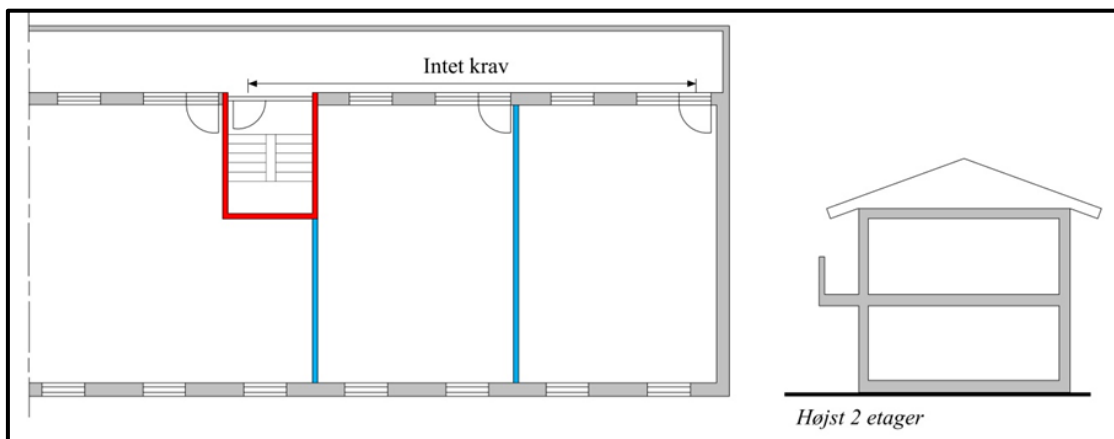
Figur 2.3.14 Adgang til flugtvejstrappe via altangang for bygning med højst 2 etager over terrænen og redningsberedskabet kan nå altangangen med deres bærbare stiger.
