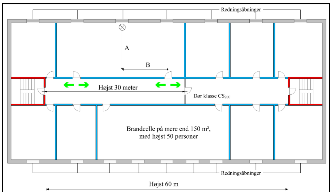
Figur 2.3.3 Døre til flugtveje fra brandceller over 150 m 2 og med højst 50 personer.
