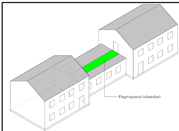
Figur 2.3.16 Flugtvej over tag til højst 50 personer.
