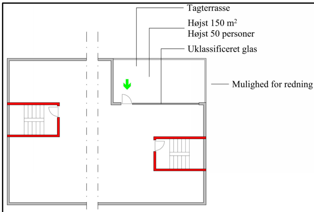
Figur 2.3.7 Flugtvej fra tagterrasse for bygninger med højst 2 etager over terræn.
