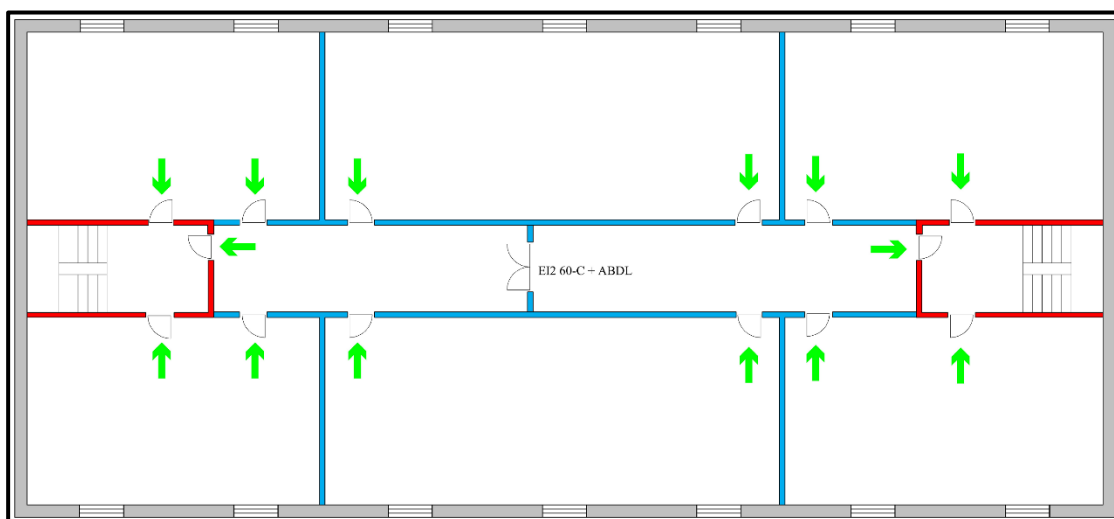
Figur 2.3.6 Opdeling af flugtvejsgang for etablering af uafhængige flugtveje fra opholdsrum.
