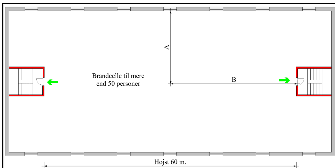
Figur 2.3.5 Døre til flugtveje fra brandcelle med flere end 50 personer, men færre end 150 personer.
