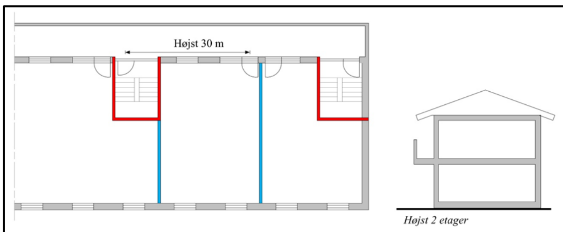
Figur 2.3.15 Adgang til flugtvejstrappe via altangang for bygning, hvor redningsberedskabet ikke kan nå altangangen med deres stiger.
