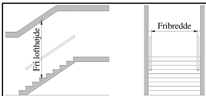
Figur 2.3.18 Definition af en trappes geometri.
