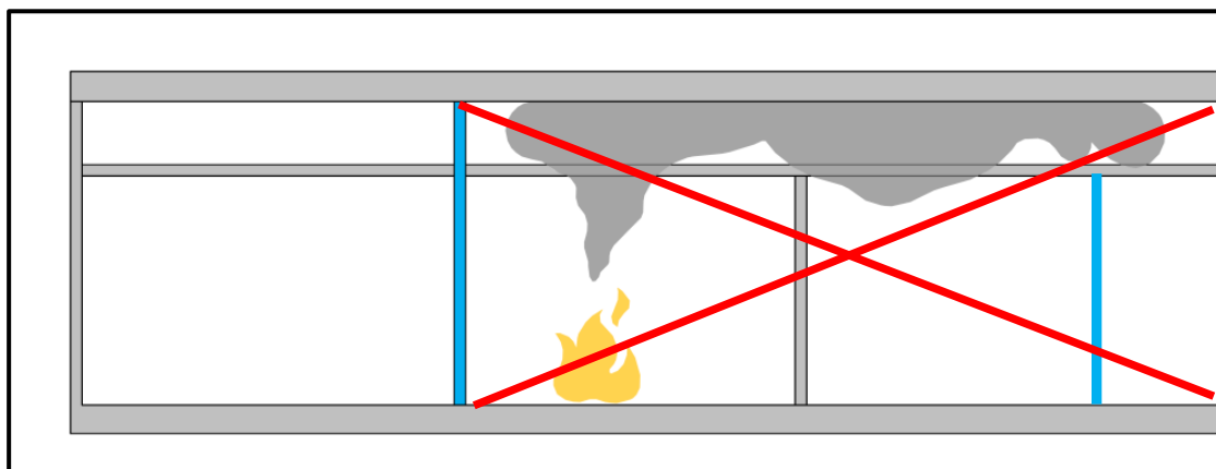
Figur 4.2.19 Brandklassificerede vægge skal føres op gennem nedhængt loft i tæt forbindelse til underside af overliggende etage eller tagkonstruktion.
