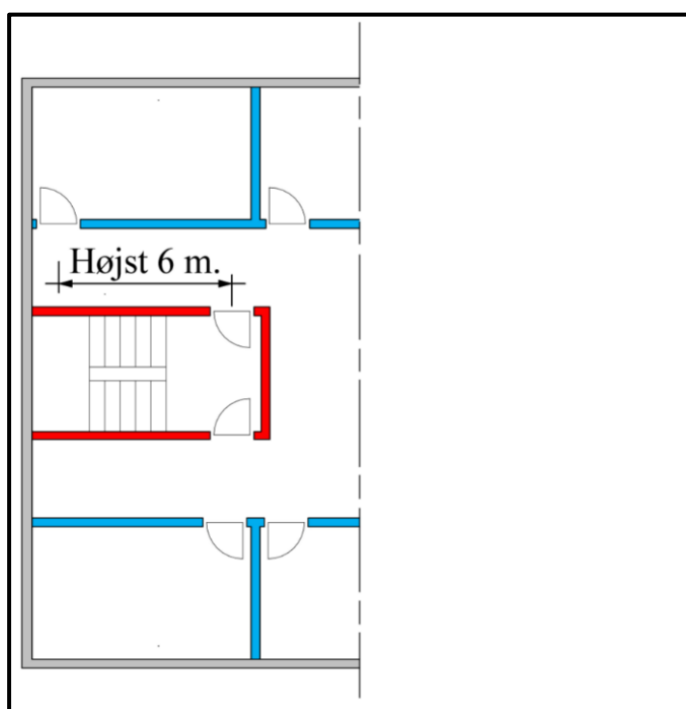
Figur 2.3.13 Udgang i én retning i en flugtvejsgang.
