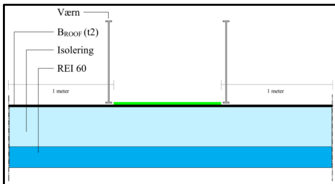
Figur 2.3.17 Brandmæssig adskillelse under flugtvej over tag. Der må ikke etableres åbninger eller gennemføringer i en afstand af mindst 1,0 m fra kanten af flugtvejen.
