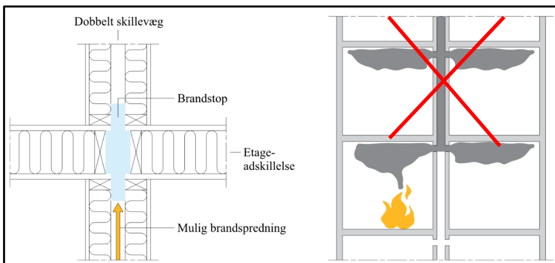
Figur 4.2.17 Brandstop mellem brandmæssige enheder.
