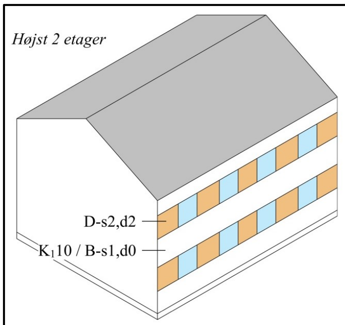
Figur 4.2.4 Præ-accepteret løsning på mindre dele af ydervæggens areal udført med regnskærm, mindst som materiale klasse D-s2,d2 [klasse B materiale]. Det samlede areal må højst udgøre 20 % af ydervæggens areal.
