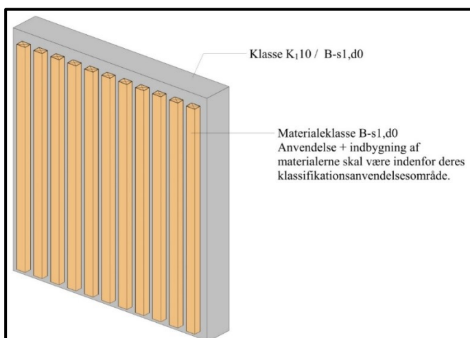
Figur 4.2.18 Præ-accepteret løsning på indvendig komplettering i form af listeværk på indvendig beklædning mindst klasse K_1 10 / B-s1, d0 [klasse 1 beklædning].
