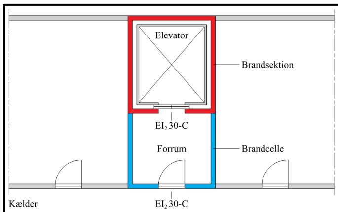
Figur 4.2.16 Adgang til kælder via forrum fra elevator.
