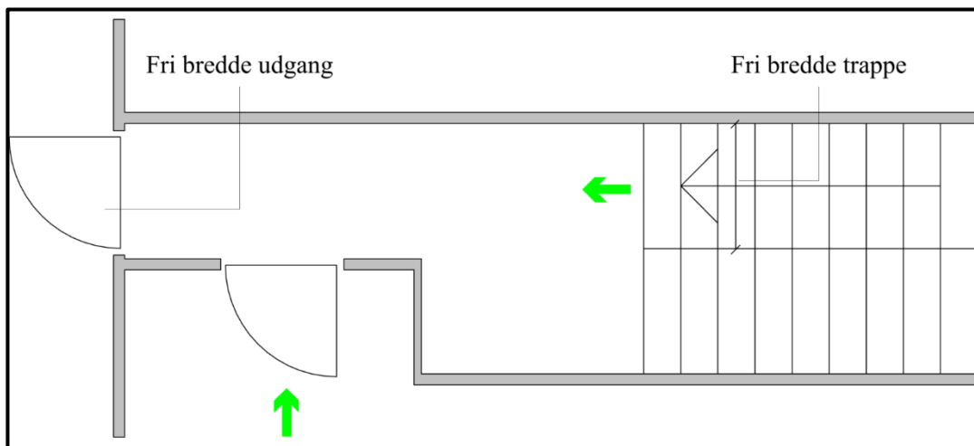
Figur 2.3.11 Fri bredde for udgang til det fri fra trapperum.
