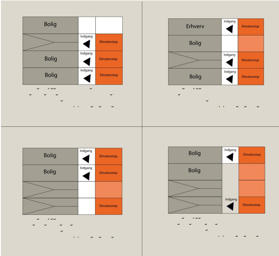
Figur 2: Eksempler på etager i bygninger (snit) - Eksemplerne er vejledende og ikke udtømmende
