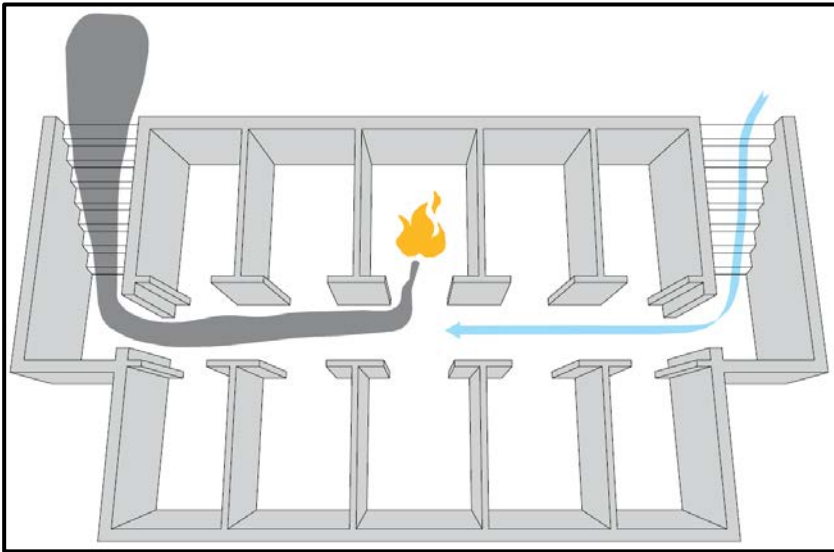
Figur 05-11-03: Eksempel på tværv ventilation
