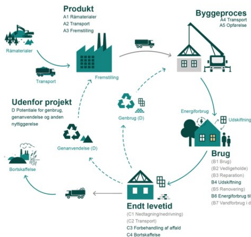
Figur 2.1: Grafisk illustration af bygningens livscyklus iht. EN15978. De moduler og faser, der indgår i beregningen, jf. § 297, er fremhævet med grøn skrift. Moduler, der ikke indgår, er markeret med grå skrift og parentes.
