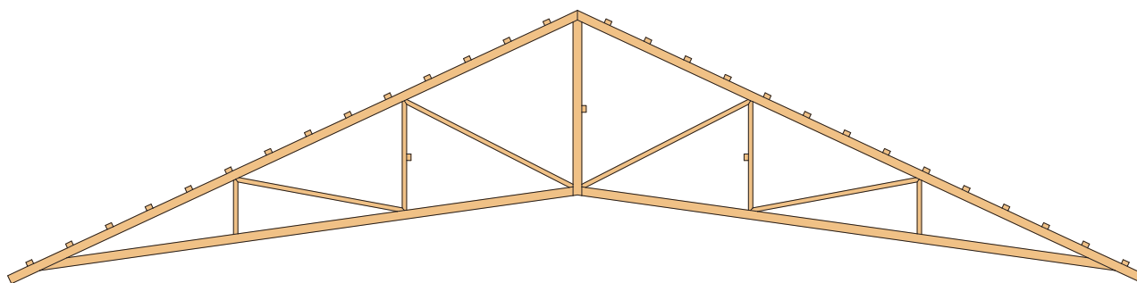
Figur 21 Saksespær har særligt store trykkræfter i spærhovederne og i de indre trykstænger.
