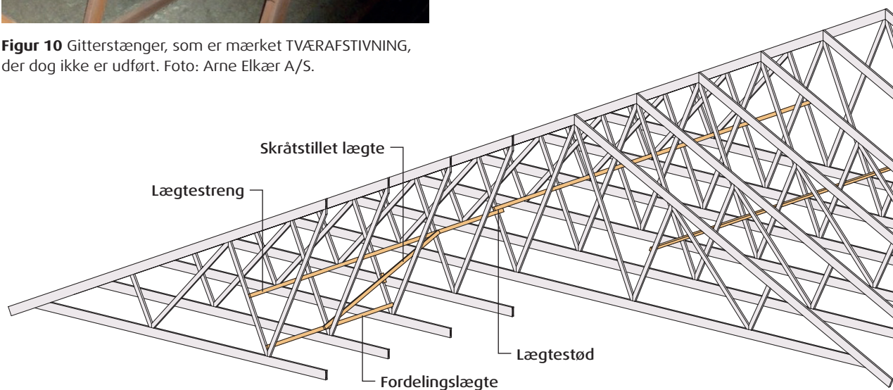
Figur 11 Gitterstænger, der er mærket med TVÆRAFSTIVNING, skal tværafstives med lægter som vist. Derudover skal lægtestrengen skråafstives med fastholdelse til loft og/eller tagflade via en fordelingslægte.
