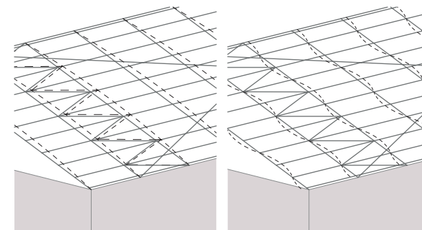
Figur 6 Eksempler på udbøjningsformer for spærhoveder, som tværafstivningen skal hindre.
