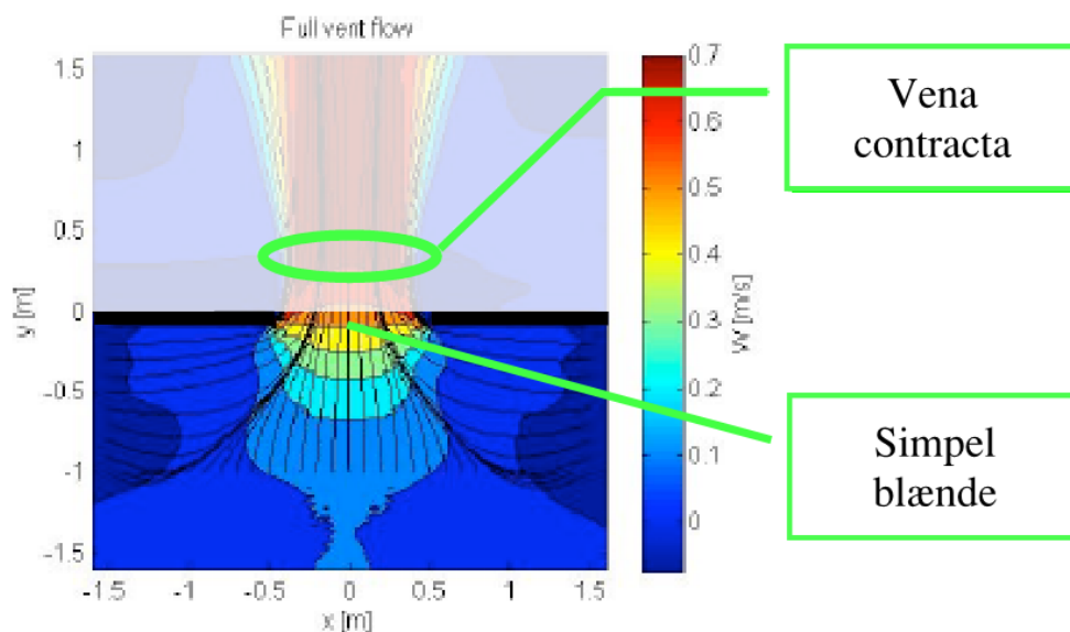
Figur 18: Simpel modellering af strømning igennem blænde uden vena contracta. Figur tilpasset ud fra CFD Best Practice [7]
