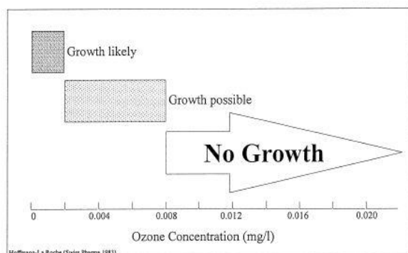
Figur 8.9. Figur viser, hvor lidt overskud af ozon i vand, der skal til, for at bakterier ikke kan overleve
