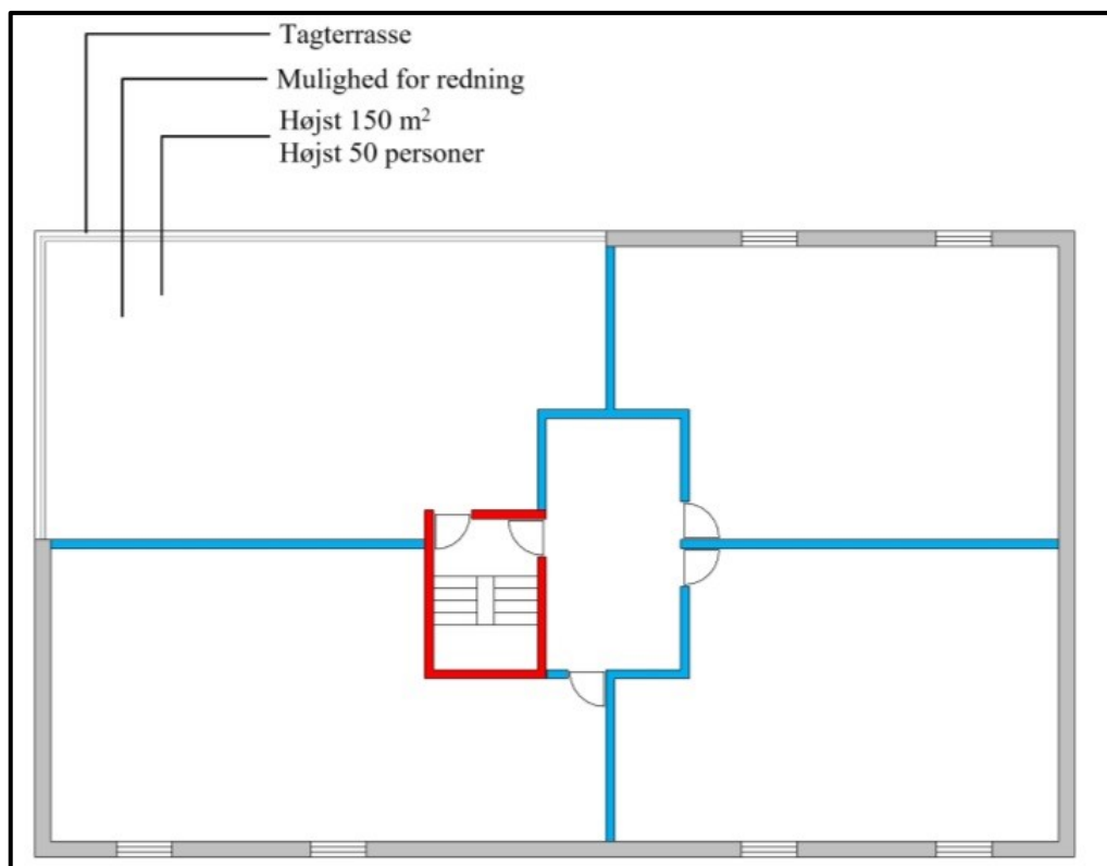
Figur 2.3.6 Flugtvej fra tagterrasse til trapperum for bygninger, hvor tagterrassens gulv er højst 22 m over terræn.
